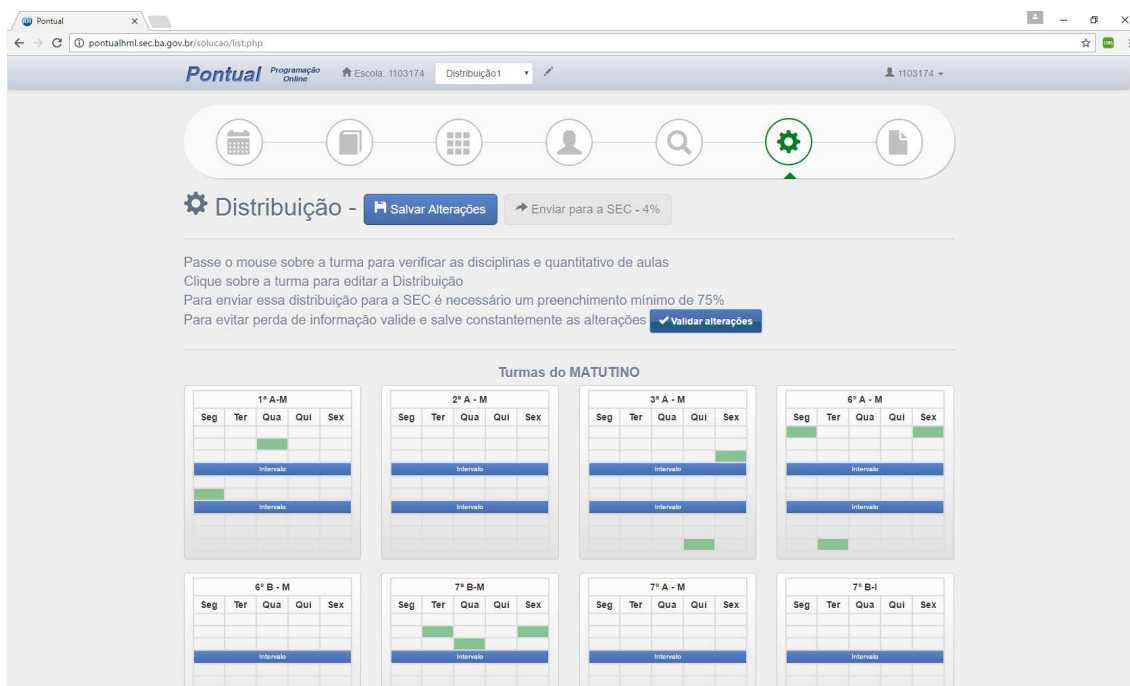
Figura 23- Exemplo de uma escola após clicar no botão de preenchimento manual e informado algumas disciplinas
