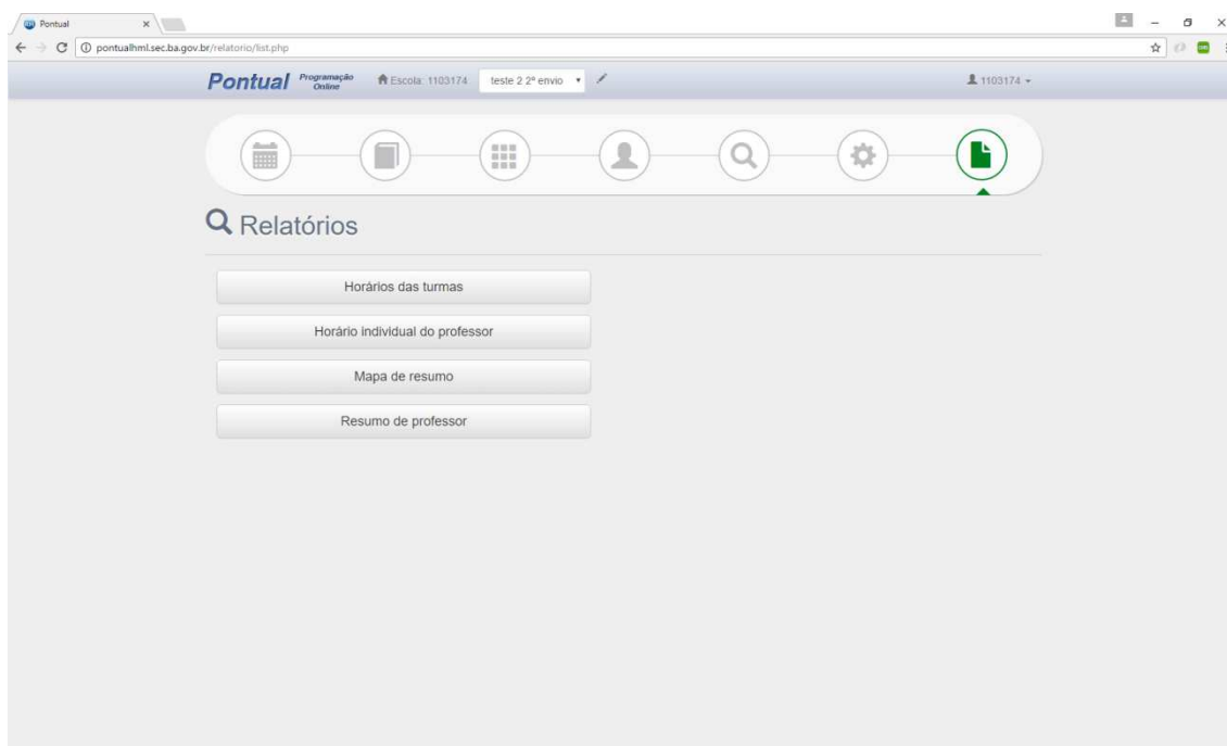
Figura 36 - Tela de listagem dos relatórios disponíveis
